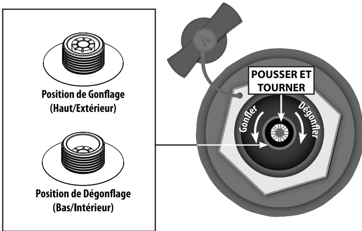
Figure 1. Gonflage/ Dégonflage Valve à ressort
