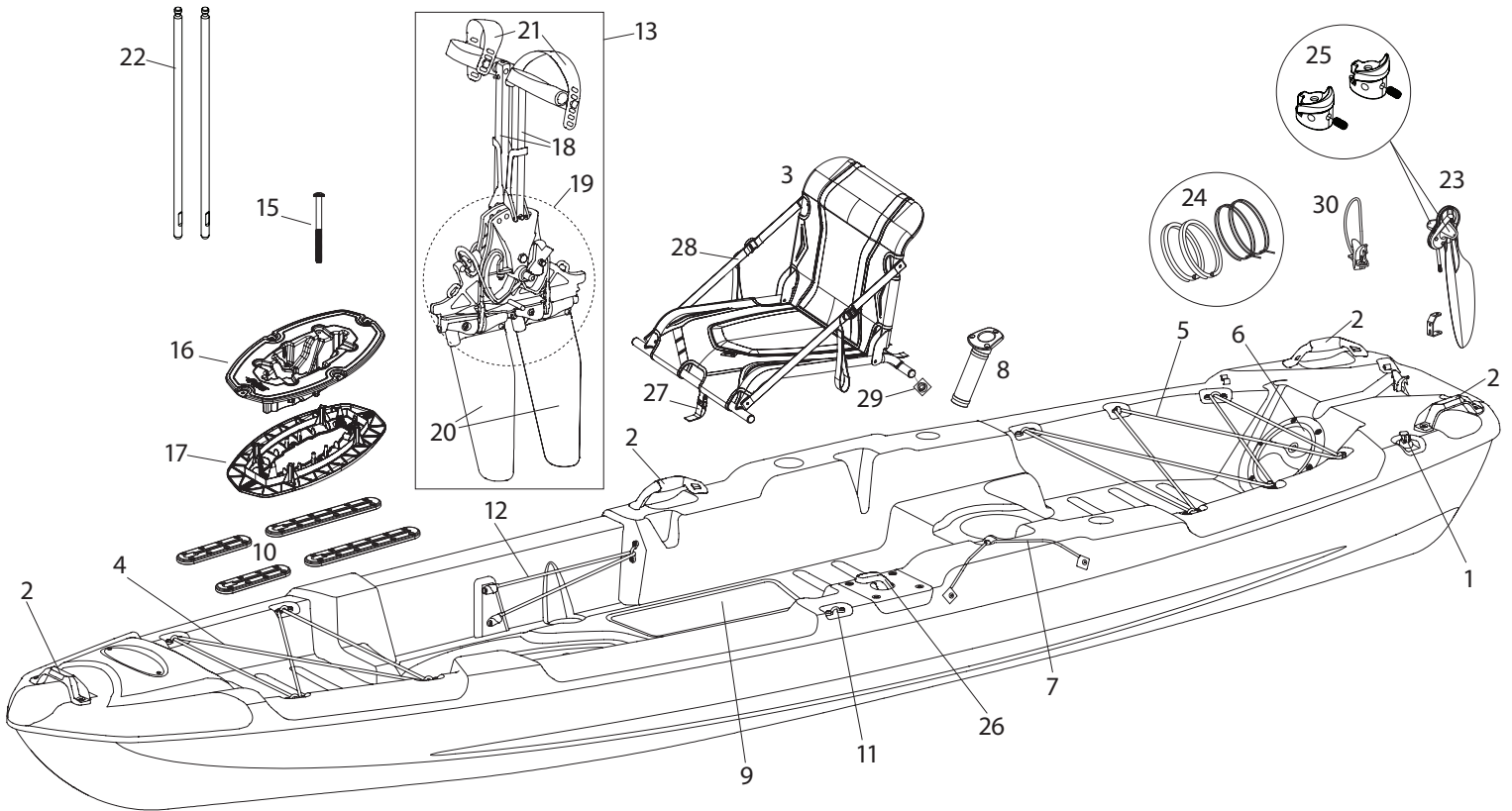
Pedal drive HYDRYVE II™ Hardware Kit - Ensemble de quincaillerie du Système d'entraînement HYDRYVE II™
