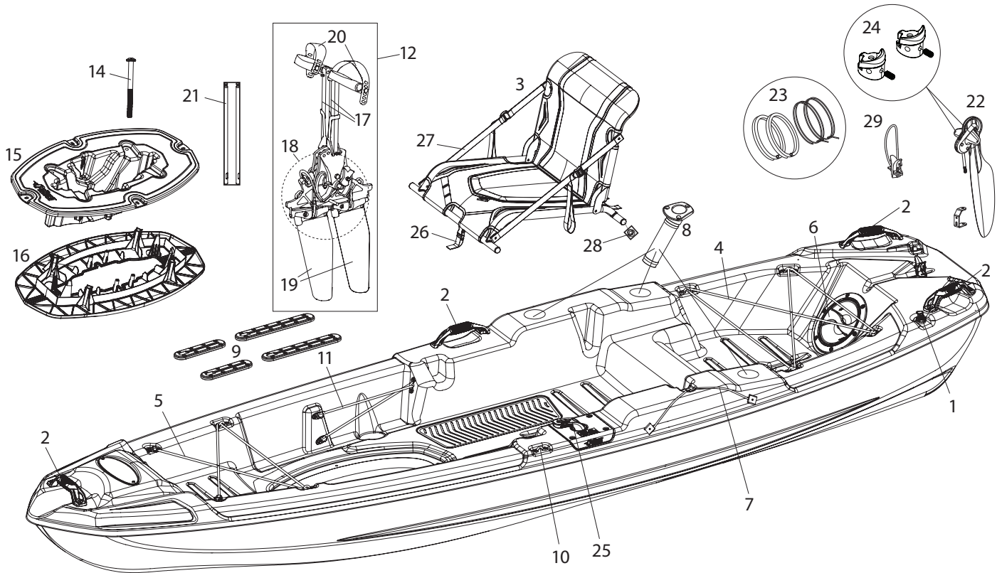
Pedal drive HYDRIVE II™ Hardware Kit - Ensemble de quincaillerie du Système d'entraînement HYDRIVE II™
